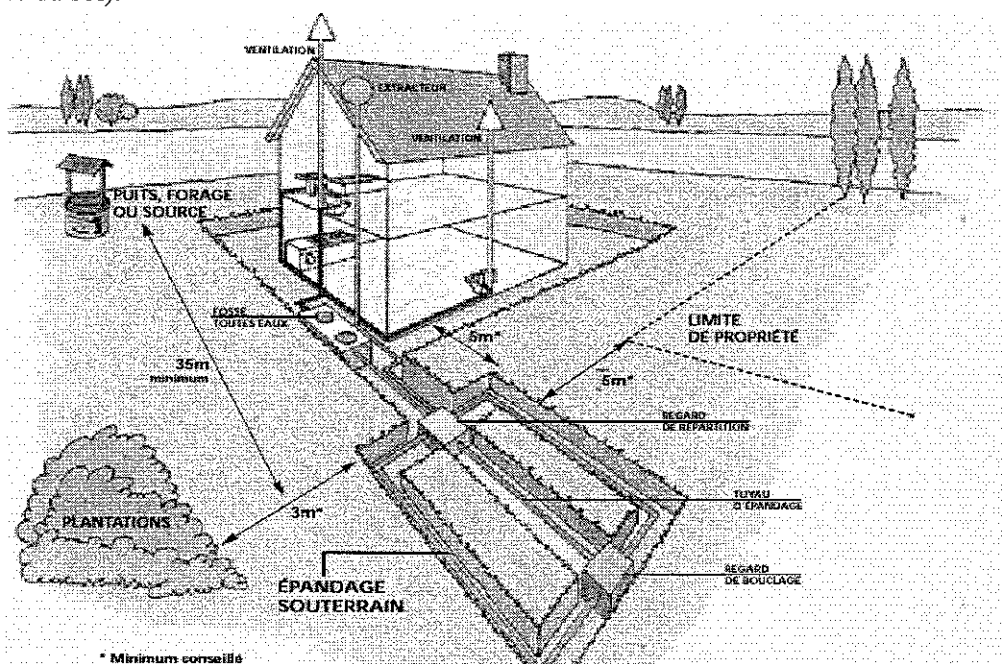
Schéma général d'un dispositif d'assainissement non collectif
