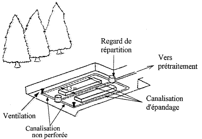
Schéma type du dispositif de traitement
