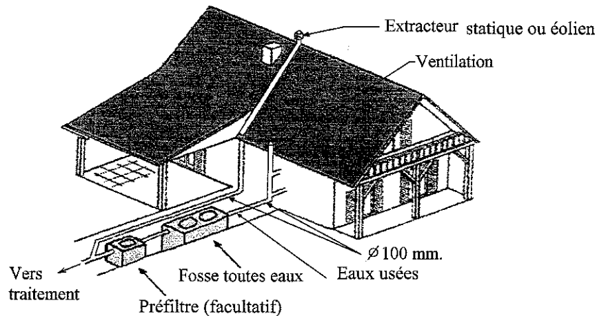
Schéma du dispositif de prétraitement
